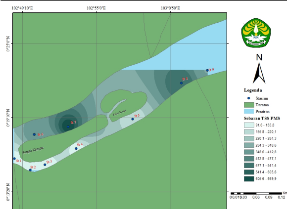
Gambar 10. Peta Sebaran Total Suspended Solid (TSS) Pasang Menuju Surut
