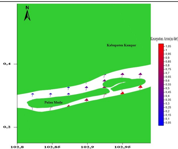
Gambar 8. Kecepatan Arus Saat Pasang Menuju Surut
