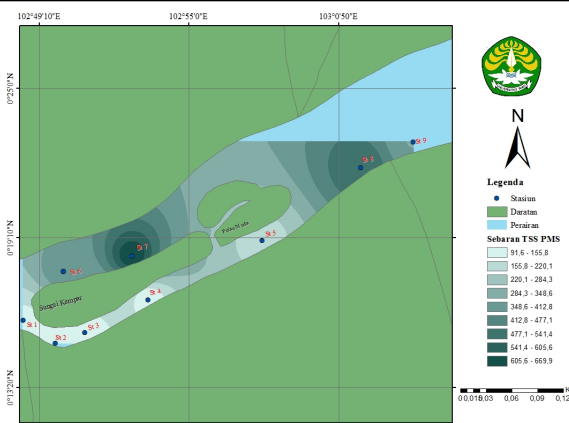
Gambar 11. Peta Sebaran Total Suspended Solid (TSS) Surut Menuju Pasang
