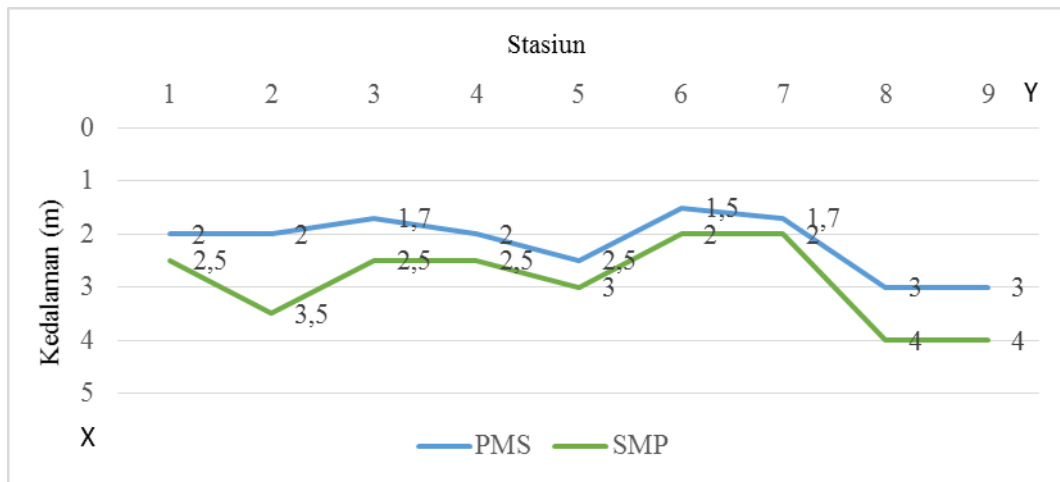
Gambar 6. Grafik Kedalaman saat Surut Menuju Pasang dan Pasang Menuju Surut
