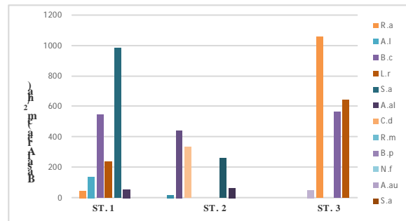
Gambar 3. Basal Area dari Setiap Stasiun
