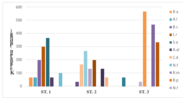
Gambar 2. Kerapatan Pohon Mangrove Setiap Stasiun
