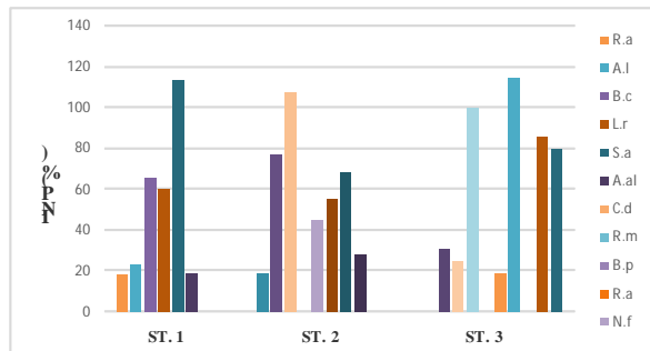
Gambar 4. Indeks Nilai Penting (%) pada Setiap Stasiun
